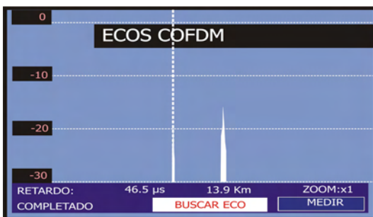
Figura 52.- Análisis de ECOS.
