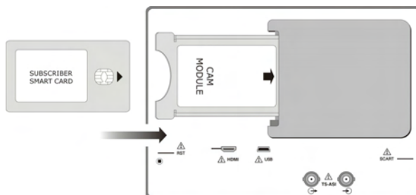
Figura 70.- Inserción de un módulo CAM y tarjeta de abonado (SMART-CARD).
