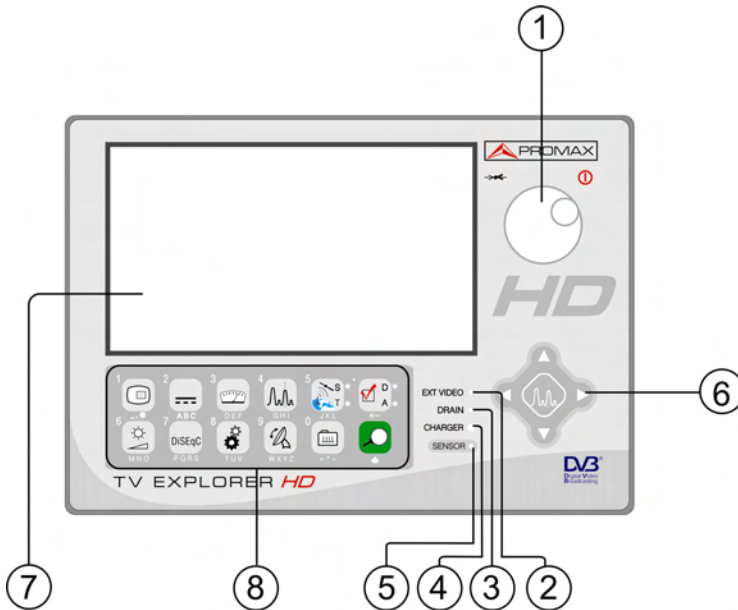
Figura 3.- Panel frontal.
