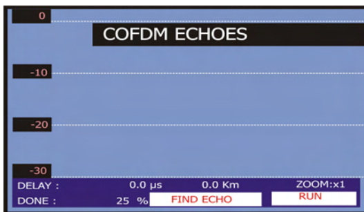
Figure 49.- Écran de la fonction ANALYSE DES ECHOS.
