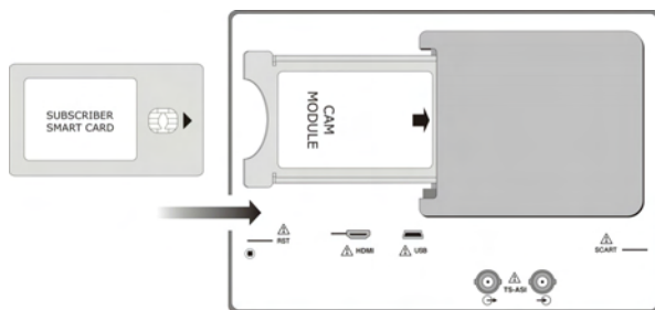
Figure 70.- Insertion d'un module CAM et carte d'abonné (SMART-CARD).
