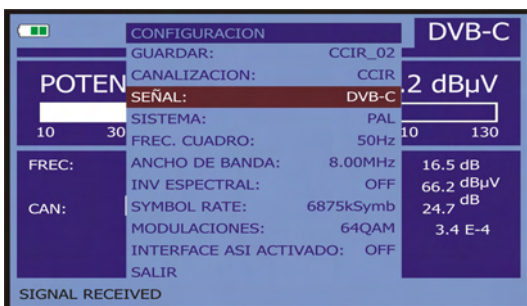
Figura 19.- Pantalla de configuración de medida de señales moduladas en QAM.
