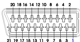
Figura 69.- Euroconector (vista externa).
