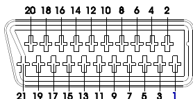
Figure 69.- Prise péritel
