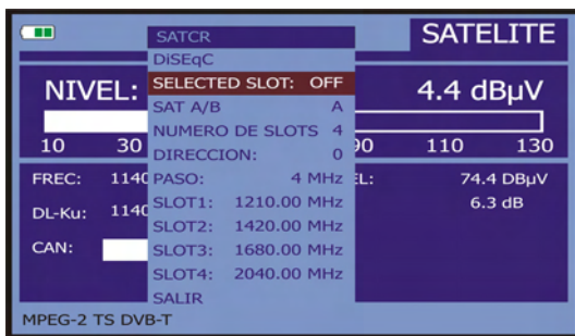
Figura 66.- Pantalla de comandos SatCR.
