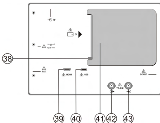
Figure 8.- Panneau postérieur.
