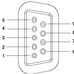
Figure 70.- Connecteur RS-232C. Raccordements vus de face.
