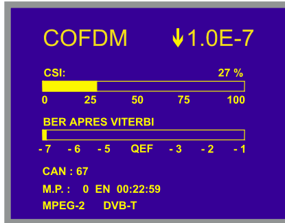
Figure 15.- Écran de mesure du BER des signaux modulés COFDM.
