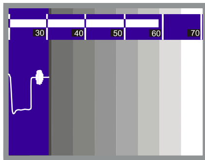
Figura 8.- Sincronismo de línea + nivel + TV (TV+NIVEL+SINC)
