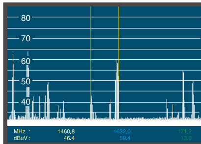
Figure 60.- Mode Analyseur de Spectres avec deux marqueurs de syntonie.
