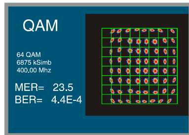
Figura 26.- Señal con niveles IQ no balanceados.
