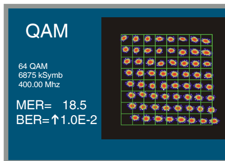
Figure 28.- Signal avec bruit et erreur de phase.
