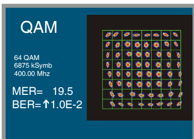
Figure 27.- Signal avec bruit et niveaux IQ non équilibrés.
