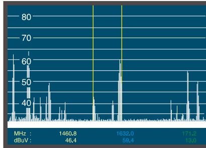
Figura 60.- Modo Analizador de Espectros con dos marcadores de sintonía.
