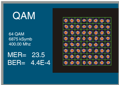
Figure 25.- Diagramme de Constellation d'un signal avec bruit.
