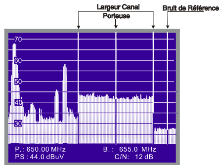
Figure 61.- Mesure C/N dans le mode Spectre (canal numérique).
