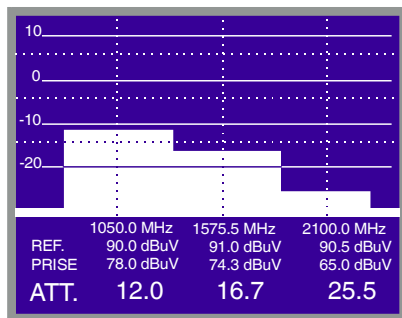
Figure 52.- Mesures d'atténuation pour une prise.
