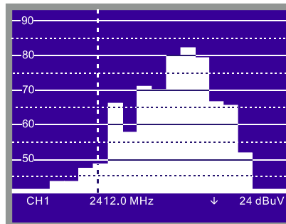
Figura 54.- Representación del espectro de la banda Wi-Fi .
