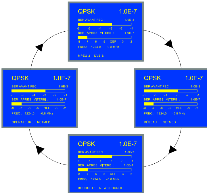
Figure 35.- Fonction DCI. Dans cet exemple, l'information codifiée par l'opérateur dans les champs Opérateur et Réseau est la même.
