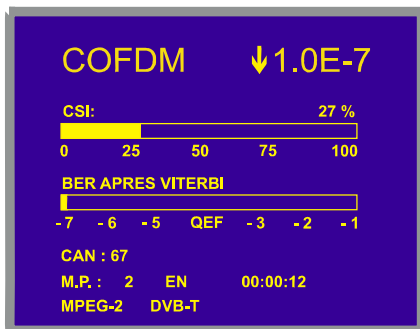
Figure 17.- Compteur RUPTURES. Dans l'exemple un total de 12 secondes sans MPEG-2 a été enregistré après 2 coupures.
