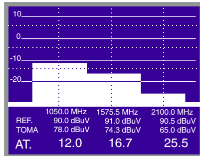
Figura 52.- Medidas de atenuación para una toma.
