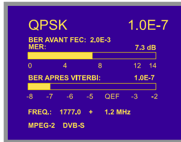
Figure 19.- Écran de mesure du BER des signaux modulés QPSK.
