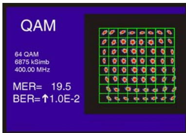
Figura 27.- Señal con ruido y niveles IQ no balanceados.
