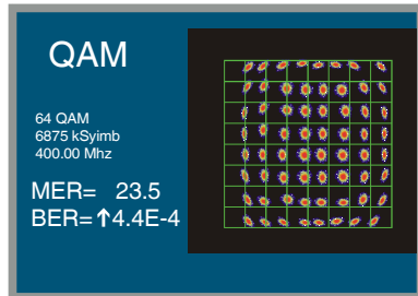
Figure 26.- Signal avec des niveaux IQ non équilibrés.
