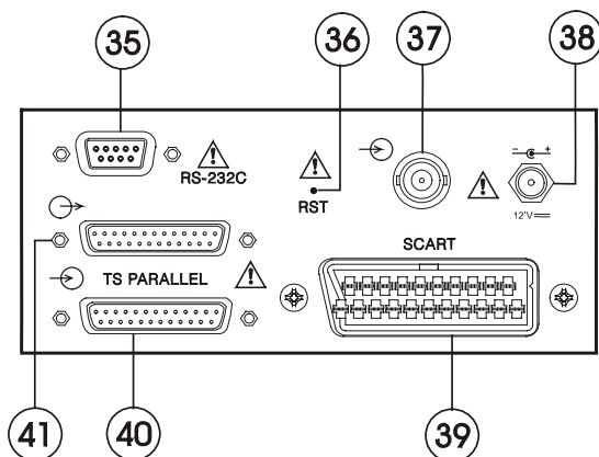
Figura 3.- Conectores del panel lateral.
