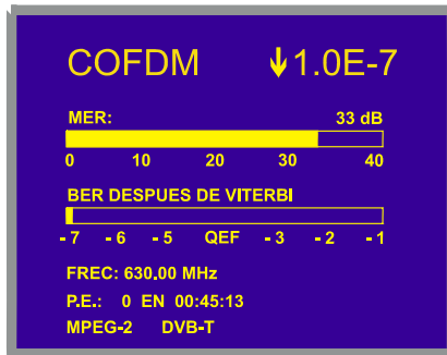
Figura 18.- Pantalla de medida del MER de señales moduladas en COFDM.
