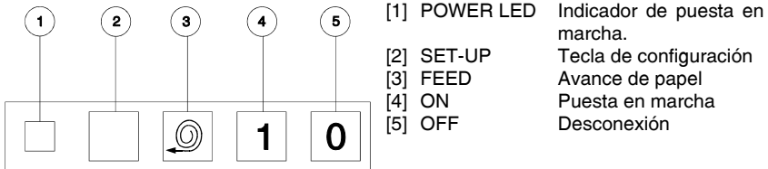
Figura 68.- Teclado impresora CI-23
