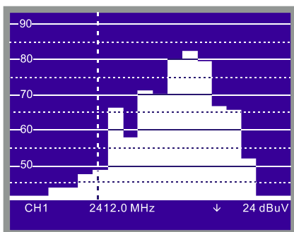
Figure 54.- Représentation du spectre de la bande Wi-Fi.
