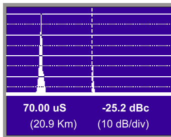
Figura 31b.- Respuesta impulsional una señal DVB-T COFDM
