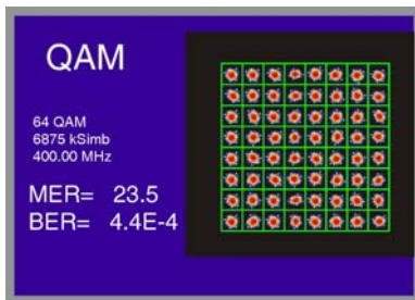
Figura 25.- Diagrama de Constelación de una señal con ruido.
