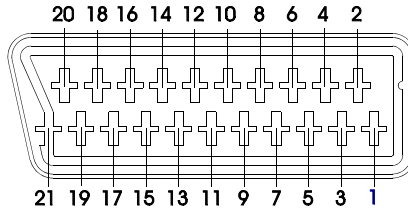
Figure 72.- Prise péritel
