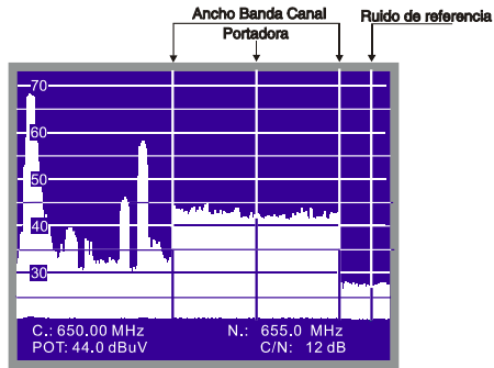
Figura 61.- Medida C/N en el modo Espectro (canal digital)
