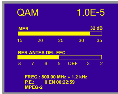
Figura 13.- Pantalla de medida del BER de señales moduladas en QAM.
