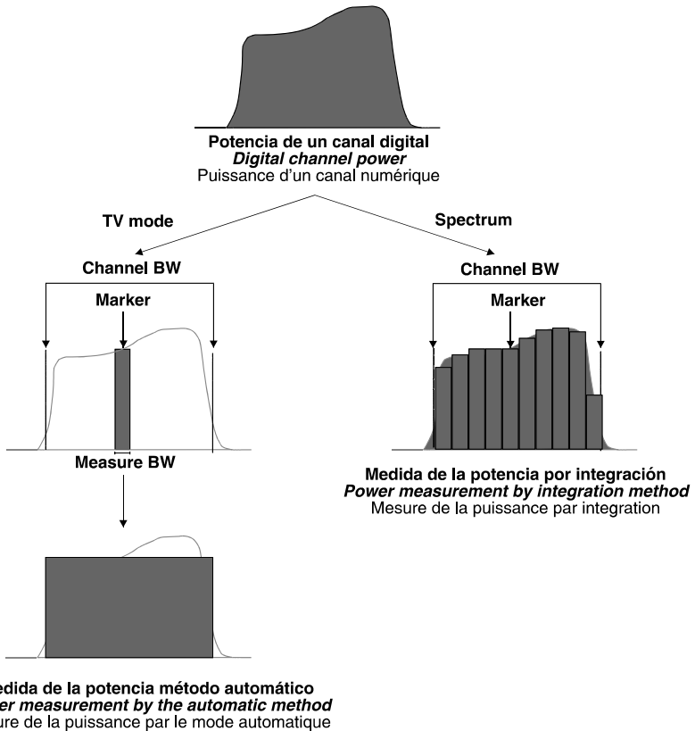
Figure 11.- Mesure de la puissance des canaux numériques.
