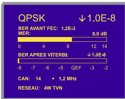
Figure 21.- Écran de mesure du MER des signaux modulés en QPSK.
