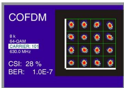
Figure 31.- Fonction Zoom COFDM.
