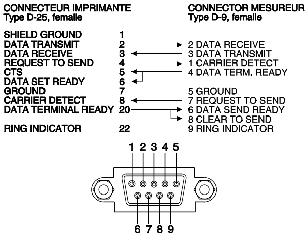
Figure 67.- PROLINK-4/4C Premium connecteur RS-232C. Numérotation des pins.
