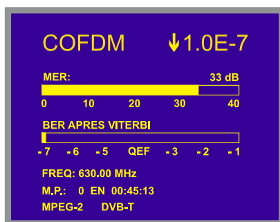
Figure 18.- Écran de mesure du MER de signaux modulés en COFDM.
