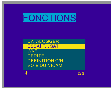
Figure 49.- Sélection de l'Essai F.I. Sat (bande satellite, mode analogique).
