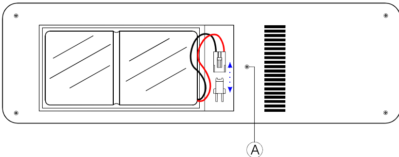
Figure 76.- Compartiment de la batterie.
