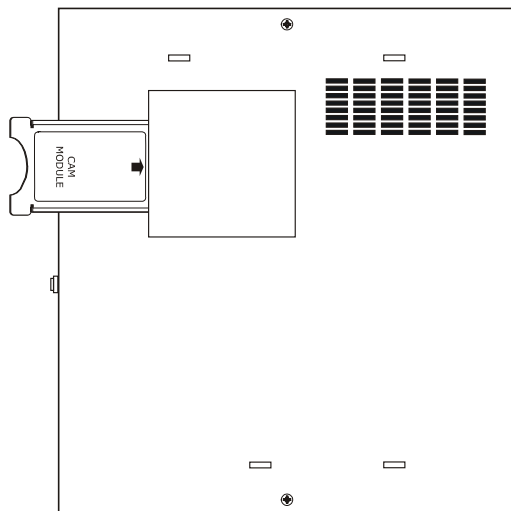
Figura 73.- Inserción de un módulo CAM.
