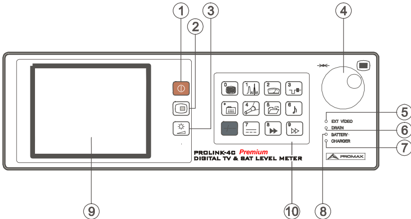
Figura 1.- Panel frontal.
