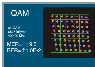
Figure 28.- Signal avec erreur de phase.
