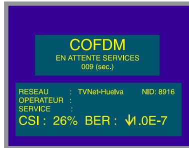
Figure 39.- Écran d'attend.
