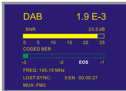
Figure 32.- Détection du signal DAB
