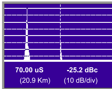
Figure 31b.- Réponse impulsionnelle d'un signal DVB-T COFDM
