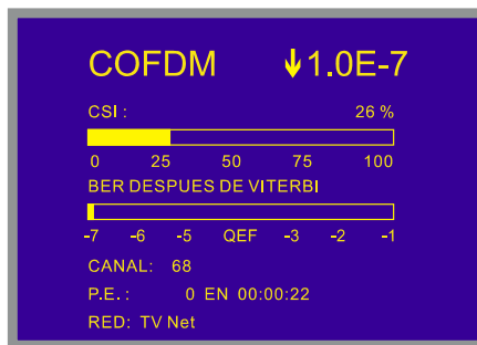
Figura 36.- Sintonización de un canal digital con nivel de BER aceptable.
