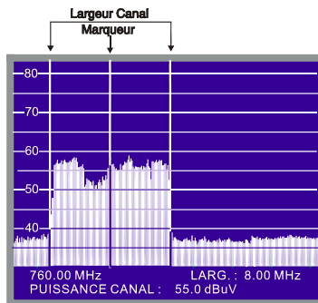
Figure 62.- Mesure de la puissance d'un canal en mode spectre.
