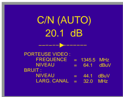
Figure 10.- Mesure du rapport porteuse / bruit C/N (mode Auto).
