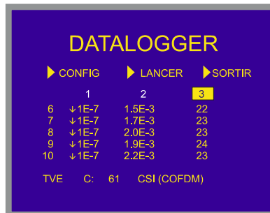
Figure 48.- Mesures automatiques des paramètres des signaux numériques.
