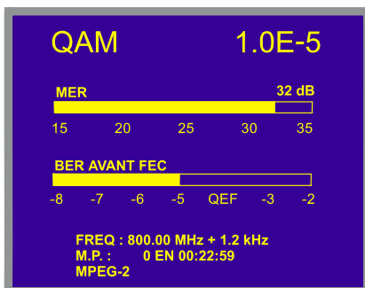
Figure 13.- Écran de mesure du BER des signaux modulés en QAM.
