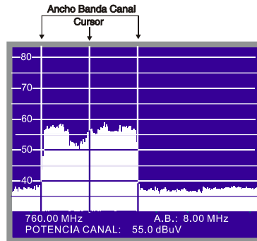
Figura 62.- Medida de la potencia de un canal en modo espectro.
