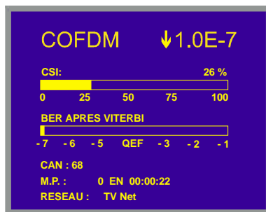
Figure 36.- Canal numérique syntonisé avec le niveau du BER acceptable.
