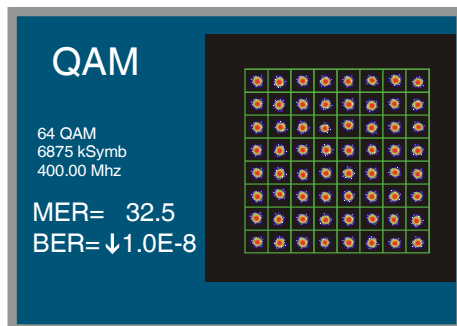
Figure 24.- Diagramme de Constellation d'un signal DVB-64 QAM correcte.
