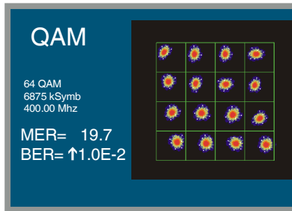
Figure 29. - Fonction Zoom QAM.
