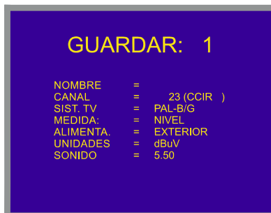
Figura 64.- Pantalla GUARDAR, almacenamiento de una configuración de medida.
