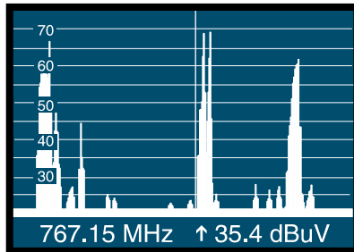
Figura 58.- Modo Analizador de Espectros
