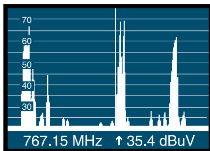
Figure 58.- Mode Analyseur de Spectres.
