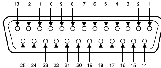
Figure 71.- Connecteur parallèle (LVDS D-25). Vue extérieure.
