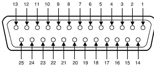
Figura 71.- Conector paralelo (LVDS D-25). Vista exterior.
