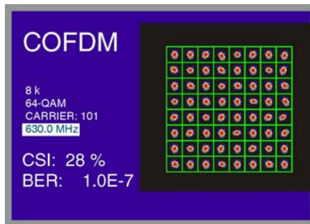
Figure 30.- Diagramme de Constellation d'un signal DVB-64 COFDM correct.
