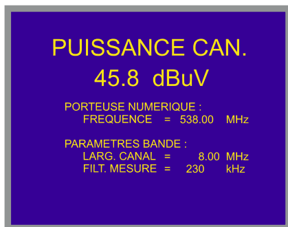
Figure 12.- Mesure de puissance des canaux numériques.
