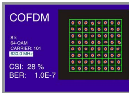
Figura 30.- Diagrama de Constelación de una señal DVB-64 COFDM correcta
