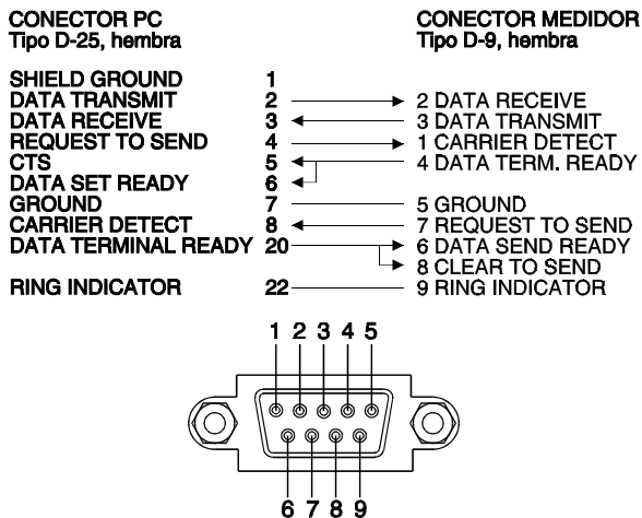
Figura 67.- Conector RS-232C PROLINK-4/4C Premium . Numeración de los pins.
