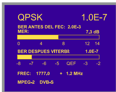
Figura 19.- Pantalla de medida del BER de señales moduladas en QPSK.
