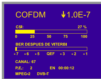
Figura 17.- Señalización de 2 cortes en la recepción de la señal MPEG con una duración total de 12 segundos.
